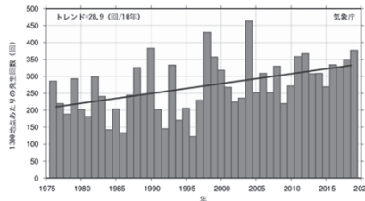
【1時間降水量50mm以上の年間発生回数】『アメダス』
